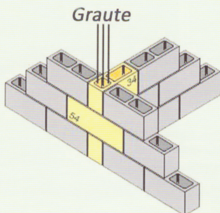
Amarração de parede em "T"
