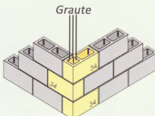
Amarração de parede em "L"
